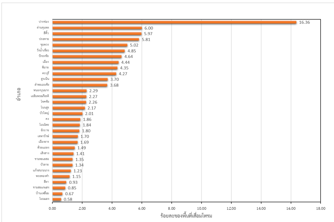
ภาพที่ 17 กราฟแสดงเนื้อที่ของพื้นที่เสื่อมโทรม รายอำเภอ จังหวัดนครราชสีมา
