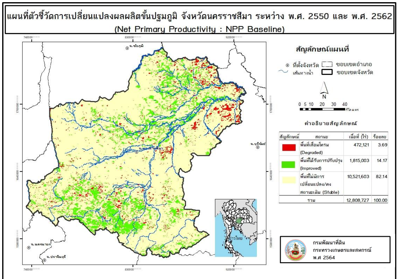
ภาพที่ 12 แผนที่ตัวชี้วัดการเปลี่ยนแปลงผลผลิตขั้นปฐมภูมิ (NPP) จังหวัดนครราชสีมา
