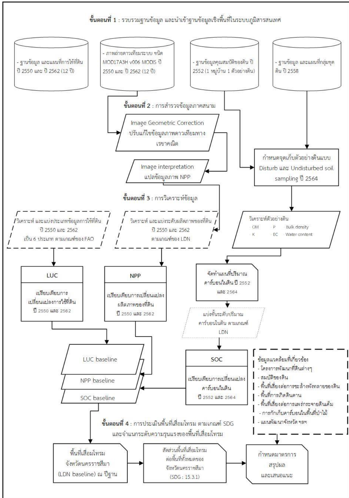
ภาพที่ 6 ขั้นตอน และวิธีการประเมินความเสื่อมโทรมของที่ดิน ตามเกณฑ์ LDN
