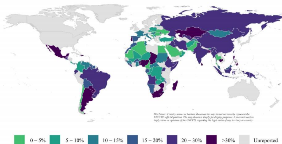
ภาพที่ 2 สัดส่วนของพื้นที่เสื่อมโทรม ในระดับโลก ตามเป้าหมายที่ 15.3.1
