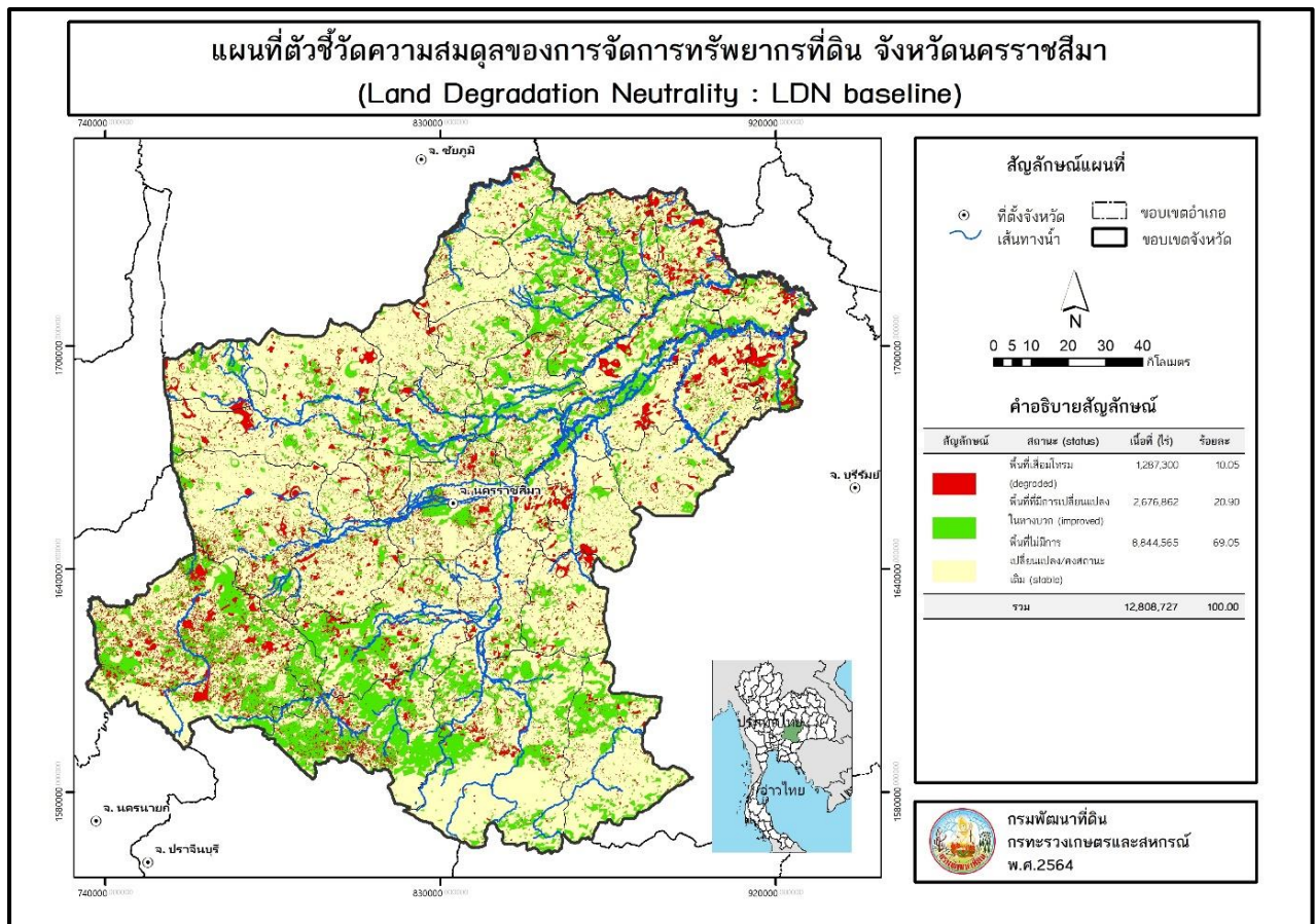
ภาพที่ 15 แผนที่ตัวชี้วัดความสมดุลของการจัดการทรัพยากรที่ดิน จังหวัดนครราชสีมา ช่วงปี พ.ศ.2550 – 2564
