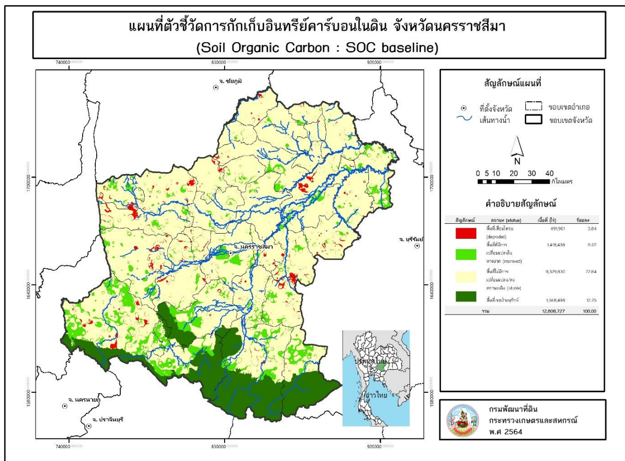
ภาพที่ 14 ตัวชี้วัดปริมาณคาร์บอนอินทรีย์ในดิน (SOC baseline) ช่วงปี 2552-2564 จังหวัดนครราชสีมา
