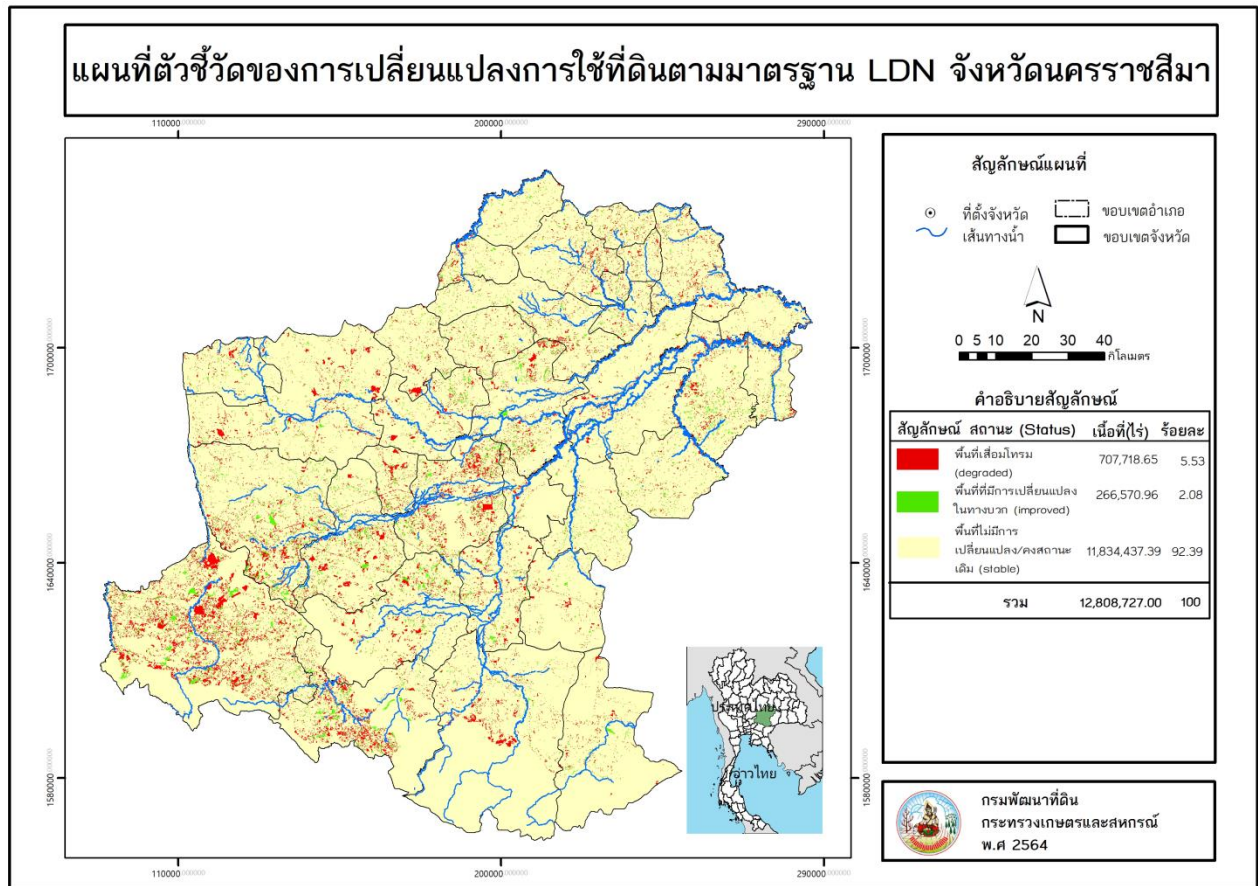
ภาพที่ 9 แผนที่ตัวชี้วัดของการเปลี่ยนแปลงการใช้ที่ดินตามมาตรฐาน LDN จังหวัดนครราชสีมา
