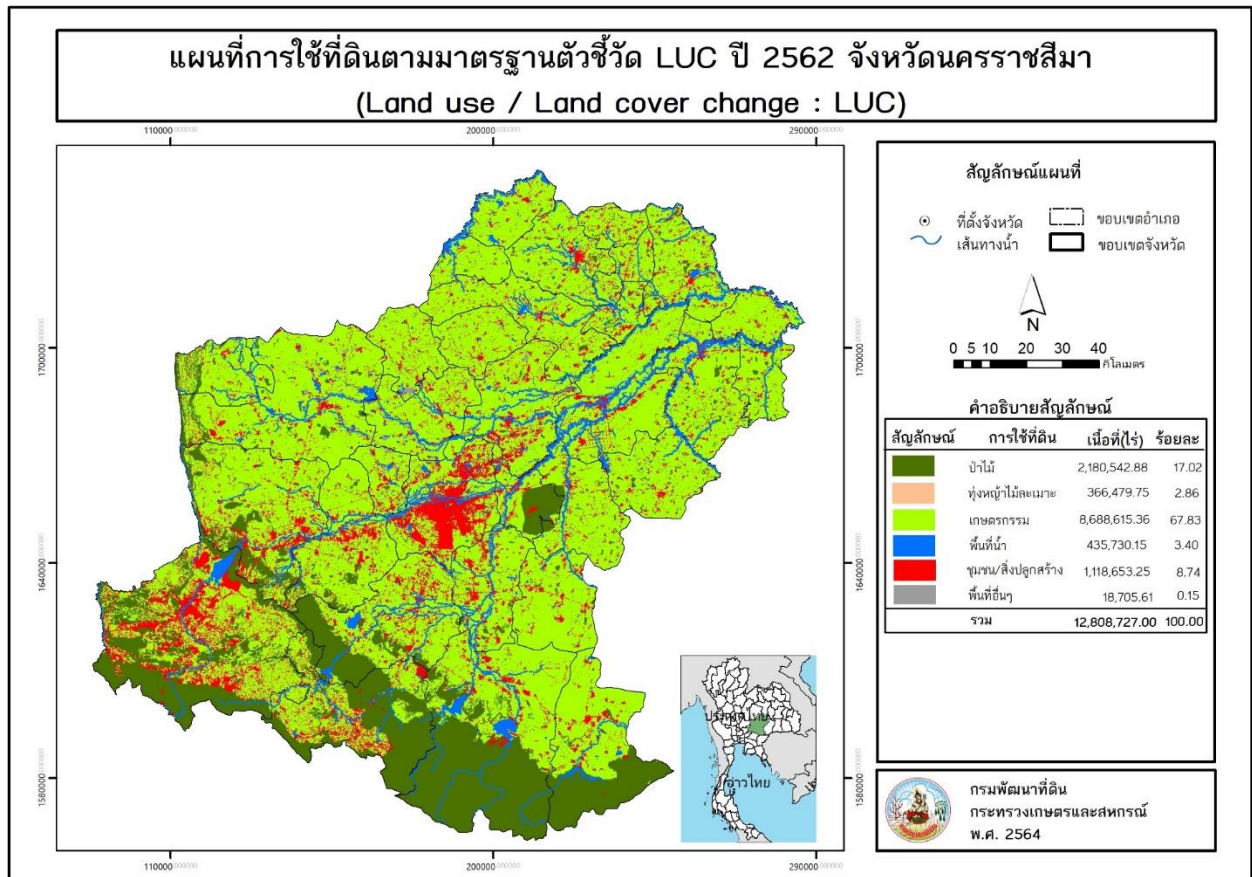
ภาพที่ 8 แผนที่การใช้ที่ดินตามมาตรฐานตัวชี้วัด LUC ปี พ.ศ. 2562 จังหวัดนครราชสีมา
