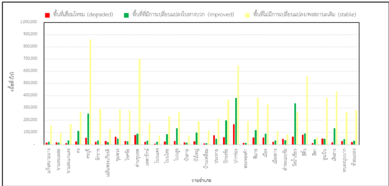
ภาพที่ 16 กราฟแสดงเนื้อที่ตัวชี้วัดความสมดุลของการจัดการทรัพยากรที่ดิน รายอำเภอ จังหวัดนครราชสีมา
